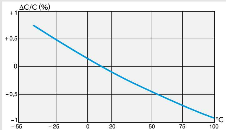
Variation relative de la capacité en fonction de la température Relative capacitance drift versus temperature
