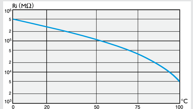
Variation de la résistance d'isolement en fonction de la température Insulation resistance change versus temperature
