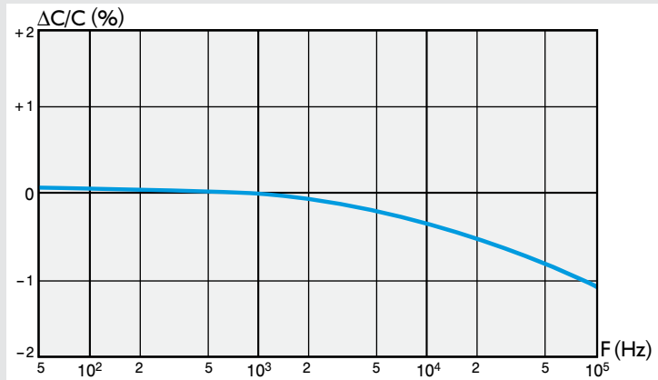
Variation relative de la capacité en fonction de la fréquence relative capacitance drift versus frequency
